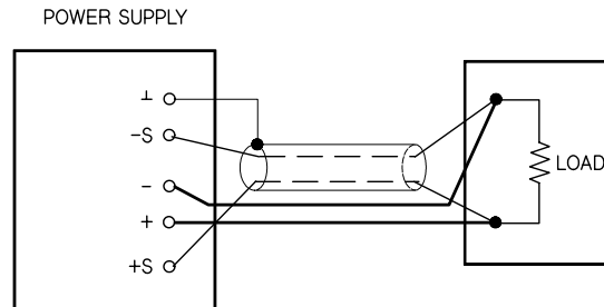
図 3-2. リモート電圧検出の接続
