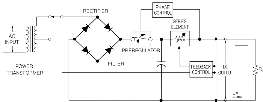
図 7-1. 直列電源装置の簡略配線図
