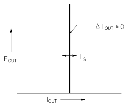
図 7-4. 理想的な定電流電源装置
