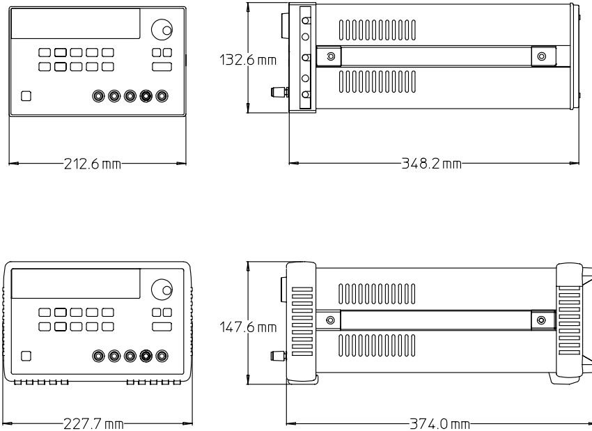
図 8-1. 電源装置 Agilent E3633A と E3634A の外形寸法
