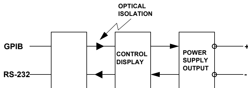
図 7-2. 光学絶縁された電源装置の構成図
