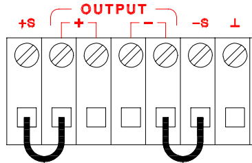
図 3-3. 背面のローカル検出接続
