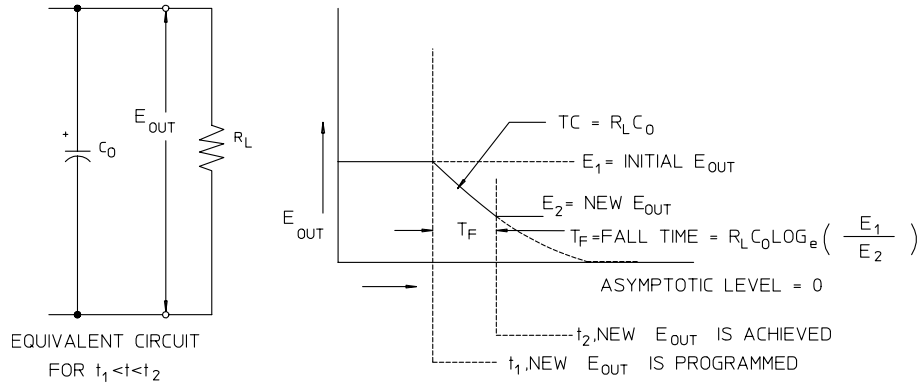
図 7-9. 応答速度 - 下降設定
