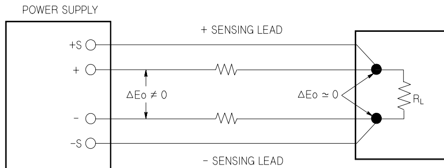
図 7-7. リモート検出機能付き調整電源装置
