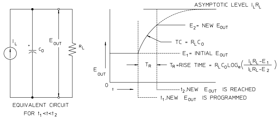
図 7-8. 応答速度 - 上昇設定 (全負荷)
