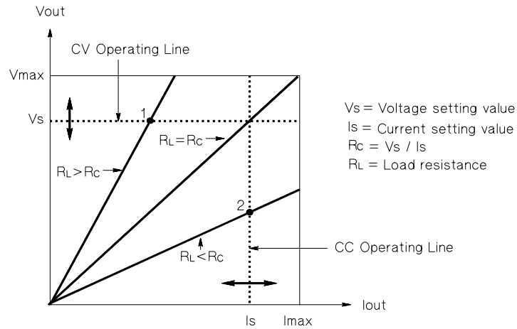
図 7-5. 出力特性
