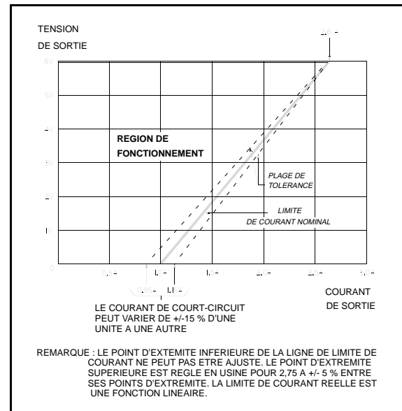
Figure 3. Caractéristique de limitation de courant de l'alimentation de 6 V
