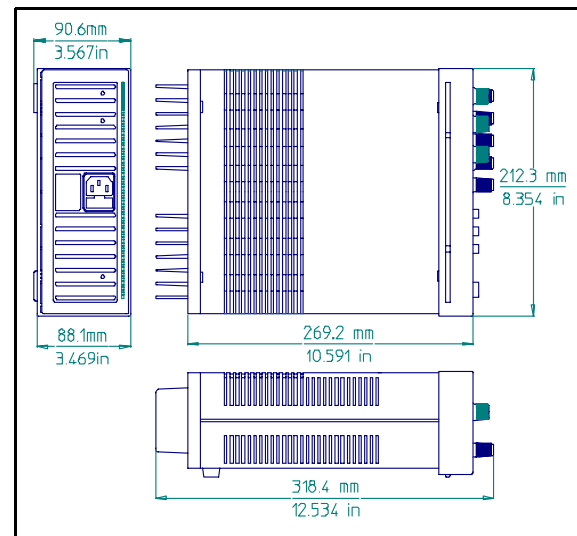
Figure 1. Schéma d'encombrement
